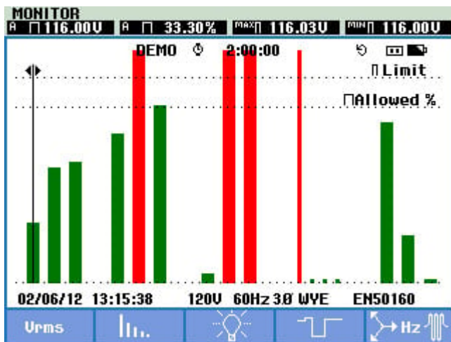
Captura de datos de onda de potencia
